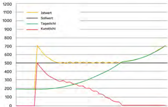
Tageslichtabhängige Steuerung im Affenhaus
